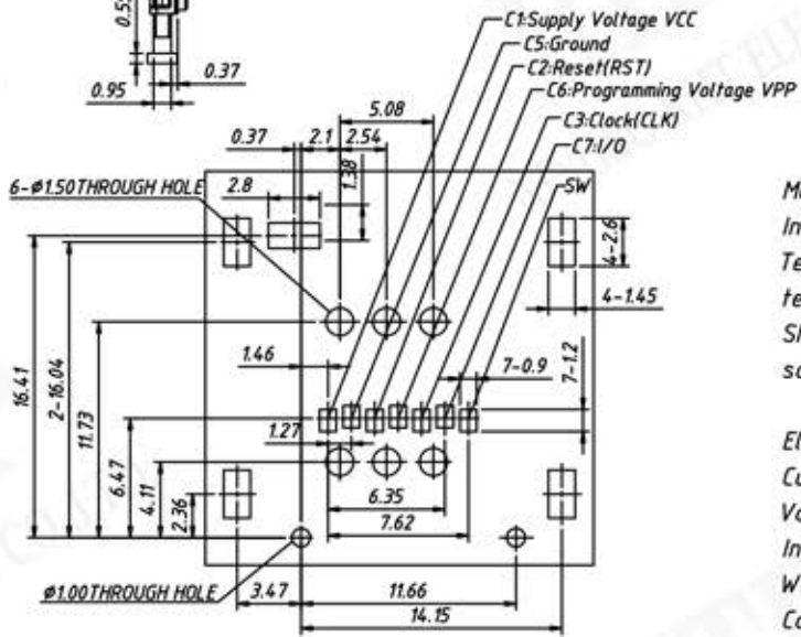
PCB LAYOUT TOL:±0.05
